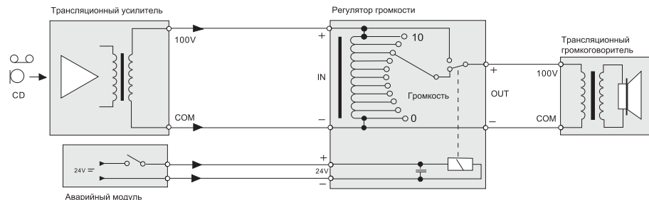
Схема подключения
