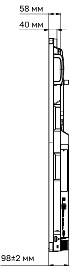
СХЕМА ПАНЕЛИ (ВИД СПРАВА)
