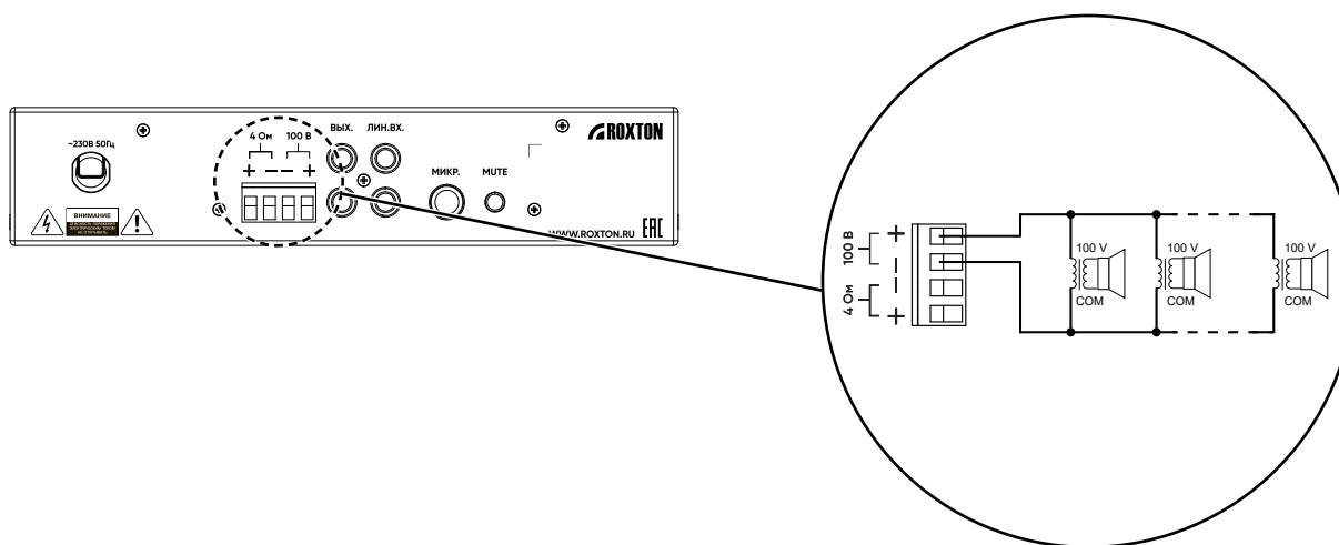
Рисунок 9.3 Схема параллельного подключения трансляционных громкоговорителей
